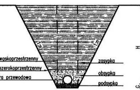
PRZEKRÓJ NORMALNY A-A
