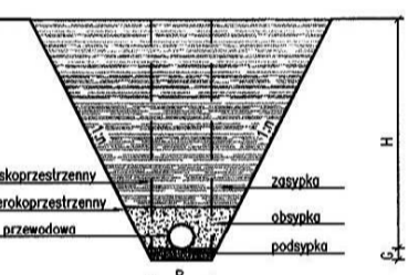
PRZEKRÓJ NORMALNY A-A
